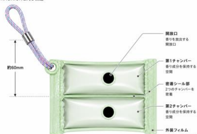
KAORION 断面図 (構造イメージ) KAORIONと同じ構造
